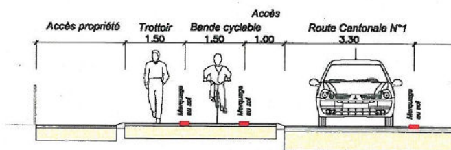
Profil d'accès à une propriété privée :
