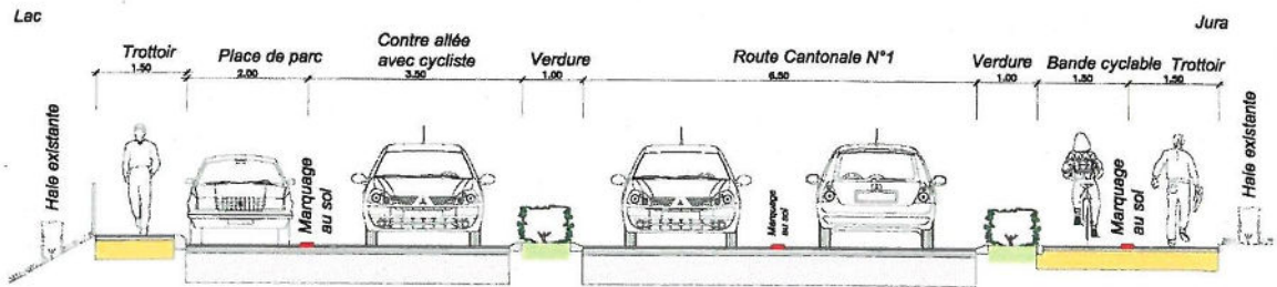
Profil chaussée avec contre-allée :
